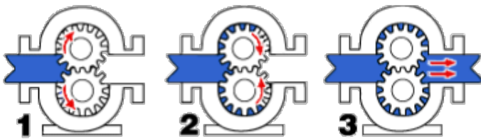
精密定量齒輪幫浦，壽命長、精度高
